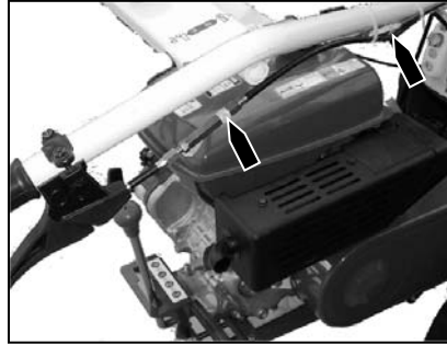
サイドクラッチ・走行ワイヤー
